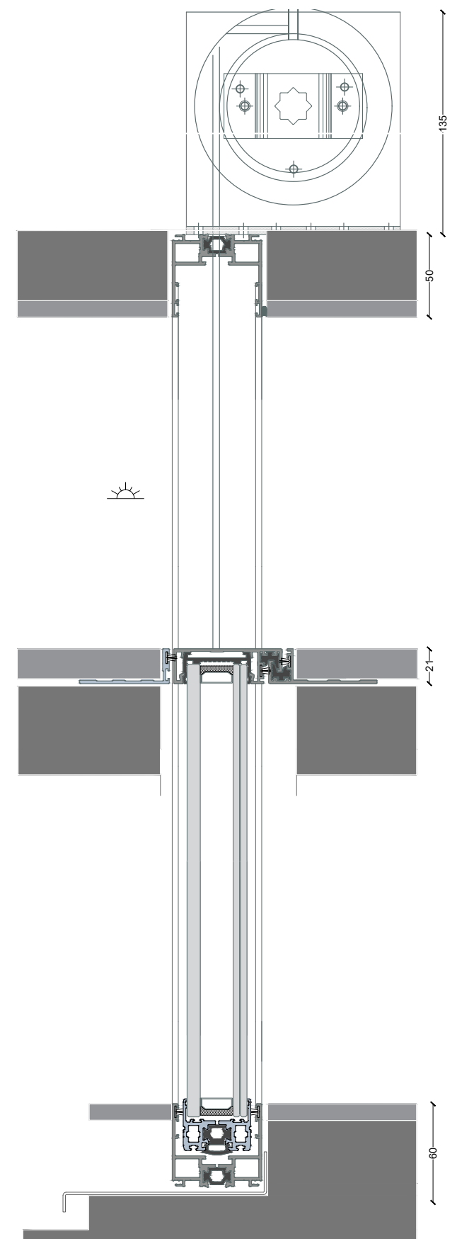
Version BAILUX G-36 1 vantail avec effacement dans le sol
