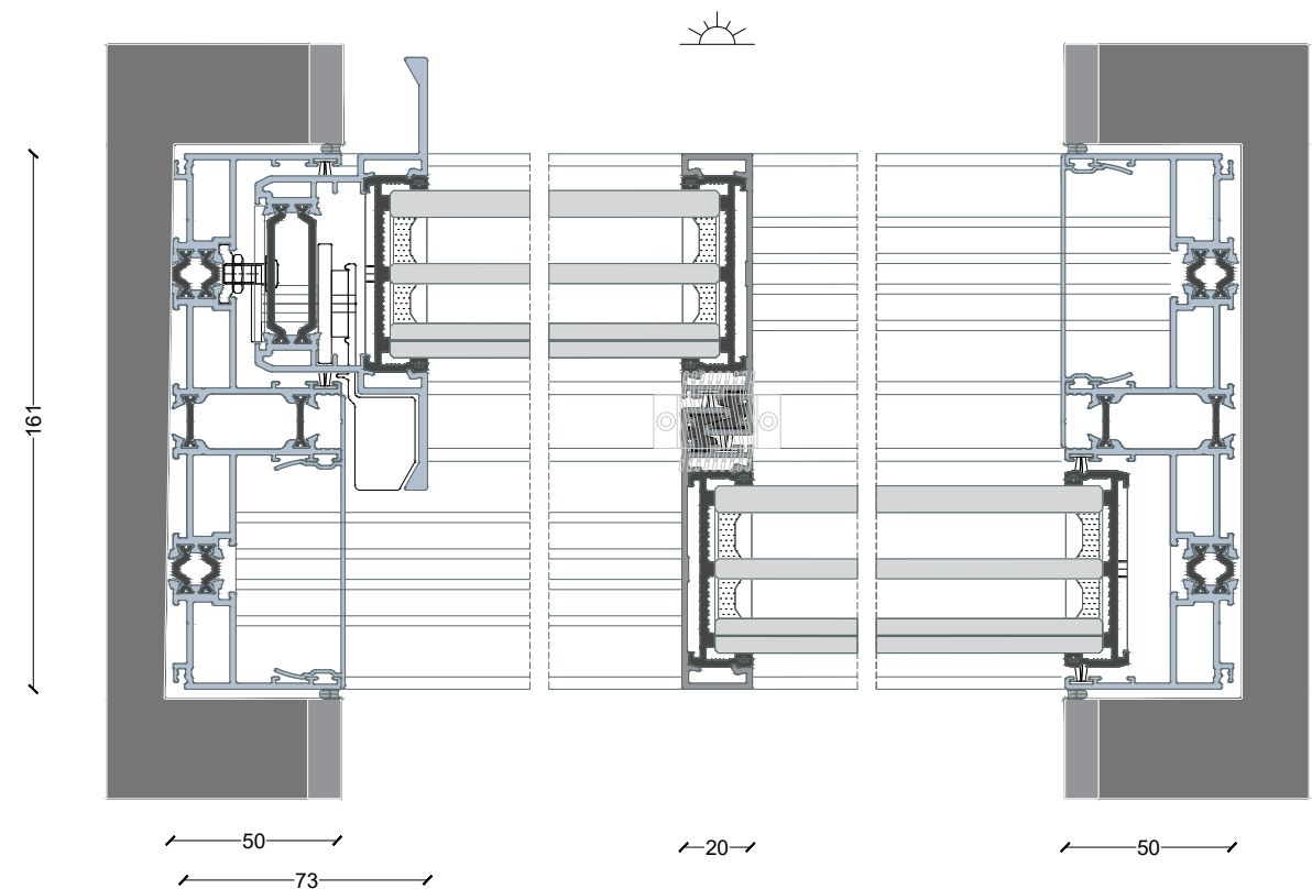
GAMME BAILUX 54 (triple vitrage)
