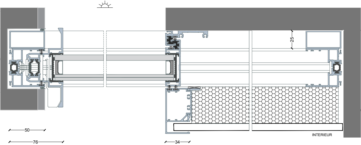
Détail variante chicane galandage
