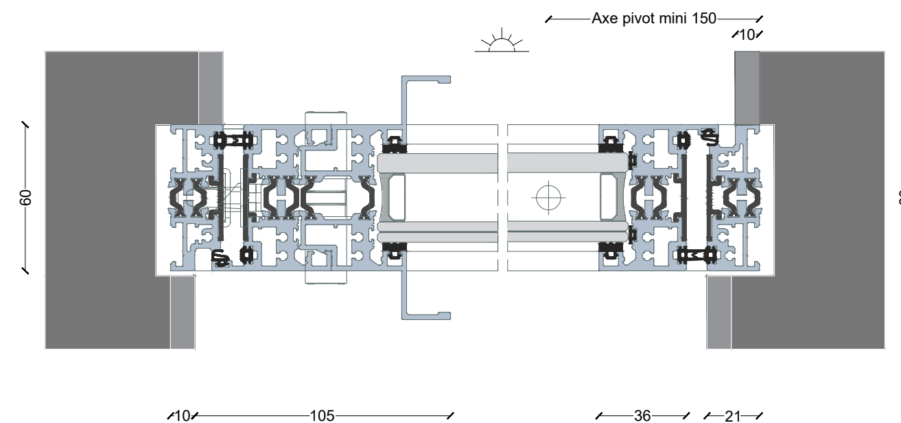
Version porte pivot sur monorail 1 vantail
